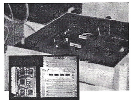
grote foto: RiscPC met 4 ARM610 RISC processoren (links achterin). Processoren mogen gemixt worden: ARM 6-, 7- en 810.
